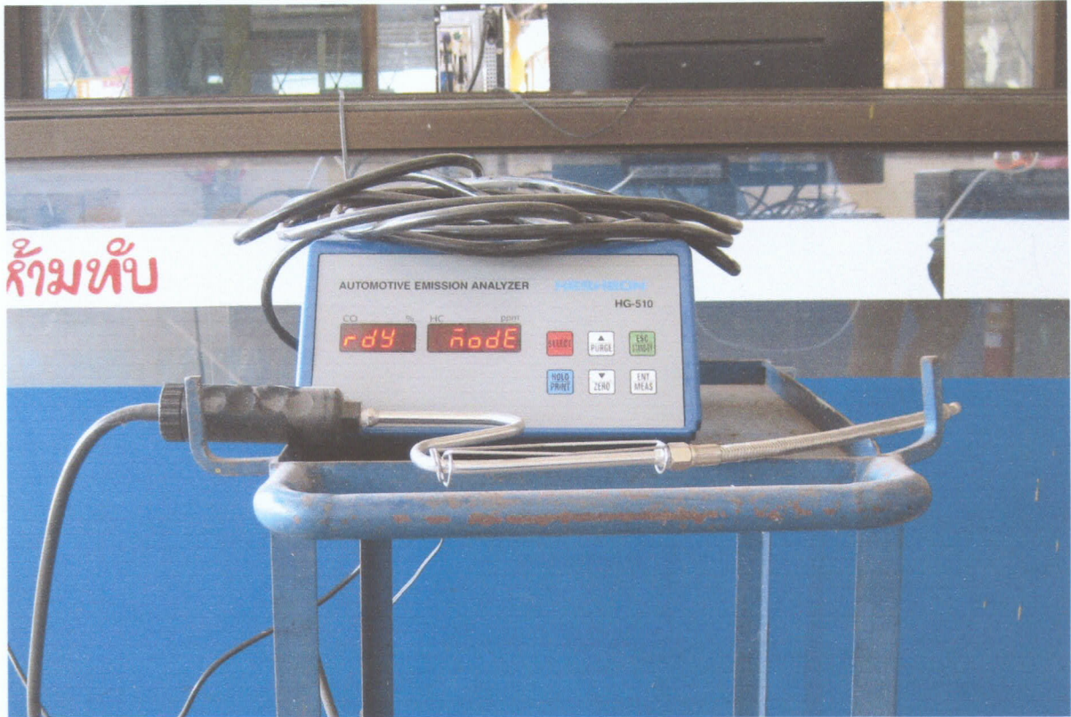
ภาพเครื่องวิเคราะห์ก๊าซ
